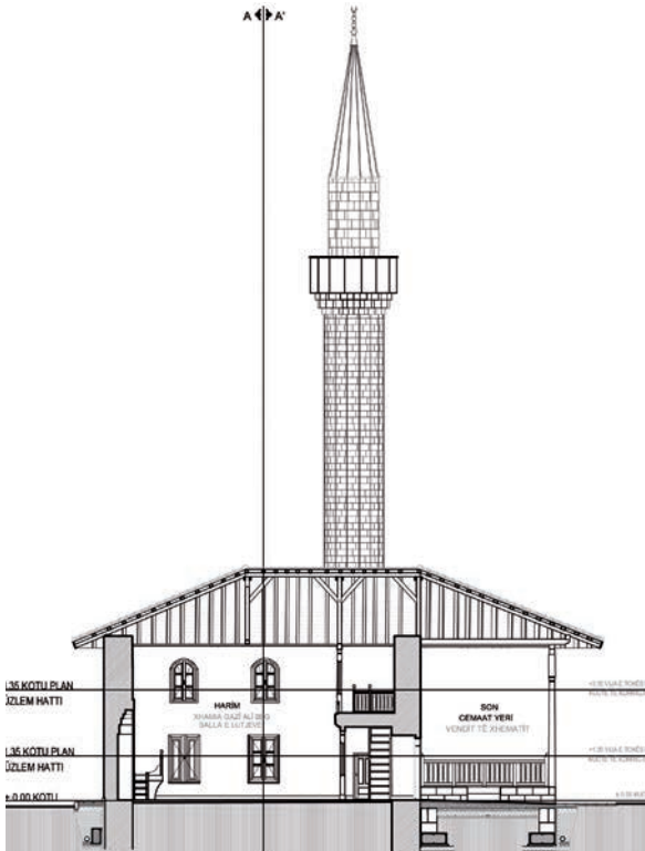
Şekil 18. Gazi Ali Bey Camii restorasyon projesi, BB kesiti (AY-MİR Mimarlık Müh. Ltd. 2015).
