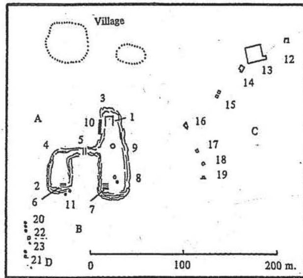
Çizim-2: Hilar Kalesi Planı (Sinclair'den)
